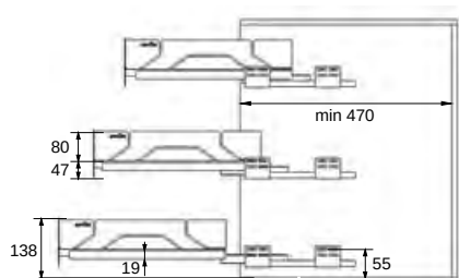
Размер базы / Base size
