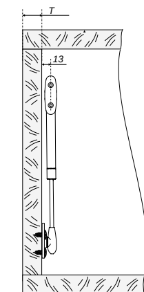
Т - наложение фасада
