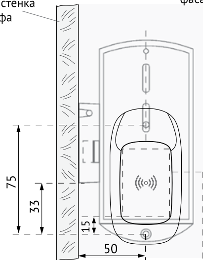
Открытие распашного фасада вправо
